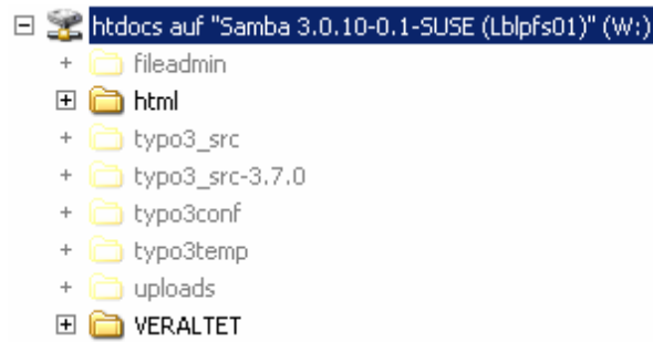
Abbildung 2: Webserver Ordnerstruktur
