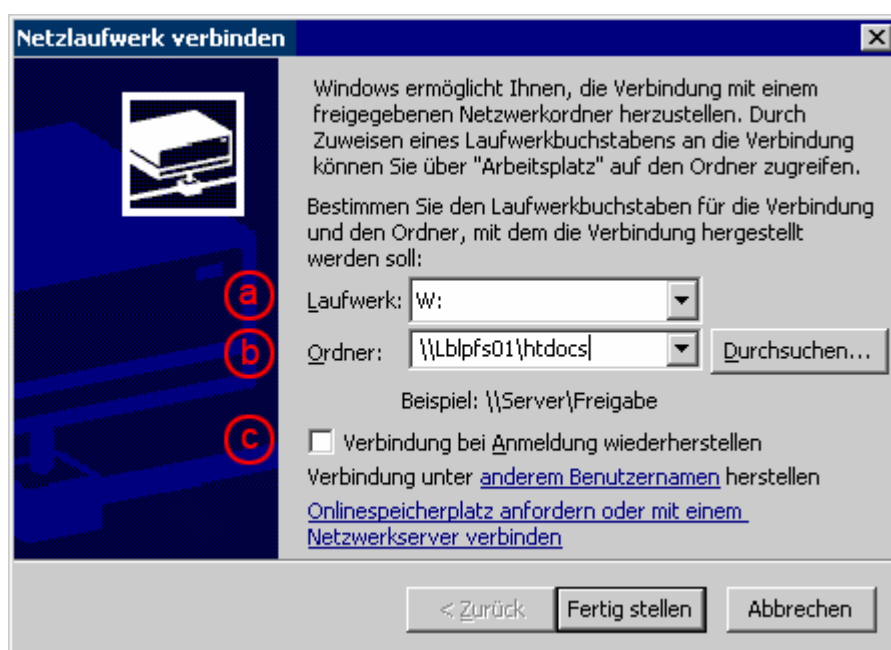
Abbildung 1: Verbindungsdialog
